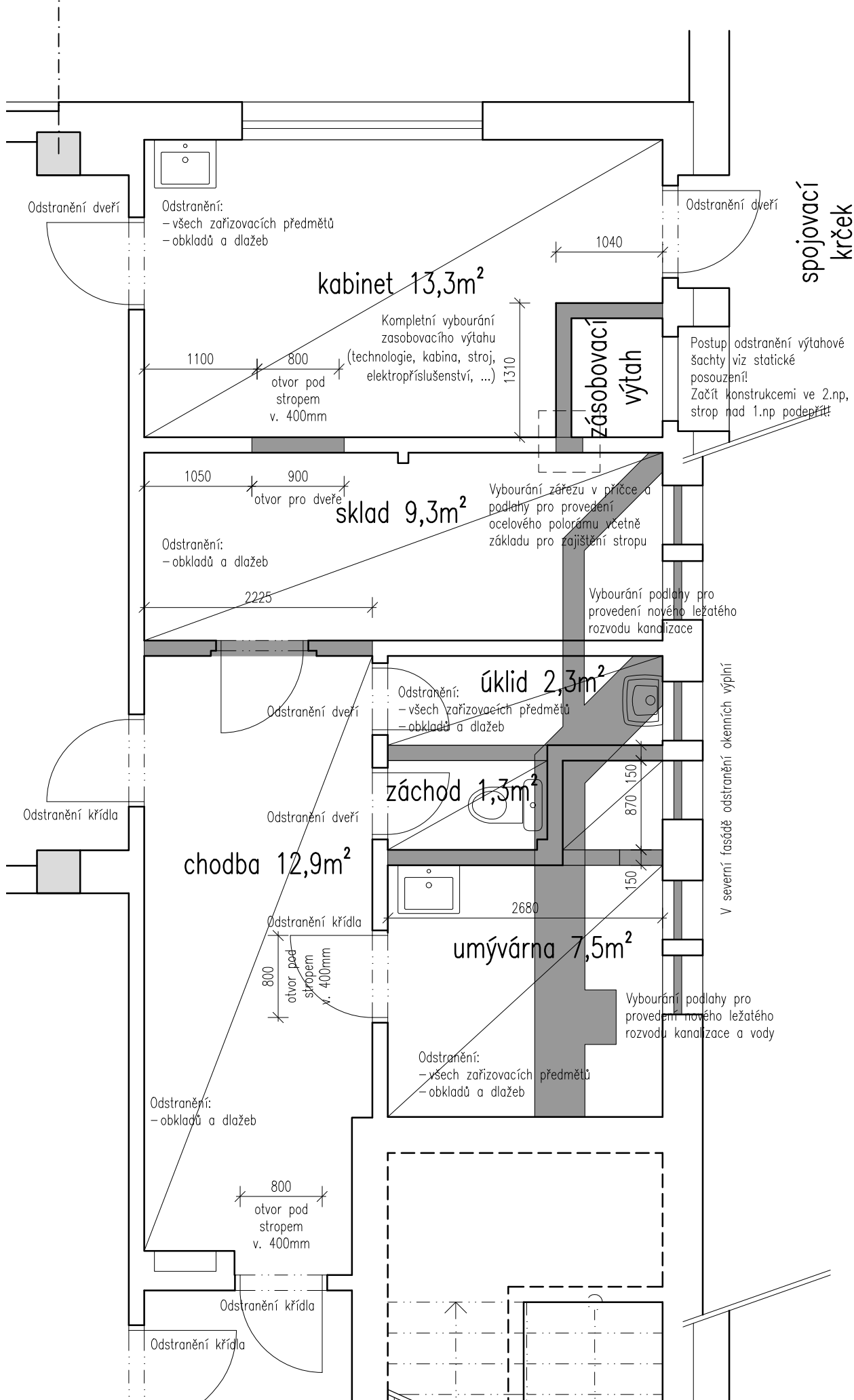
Půdorys 1.np
