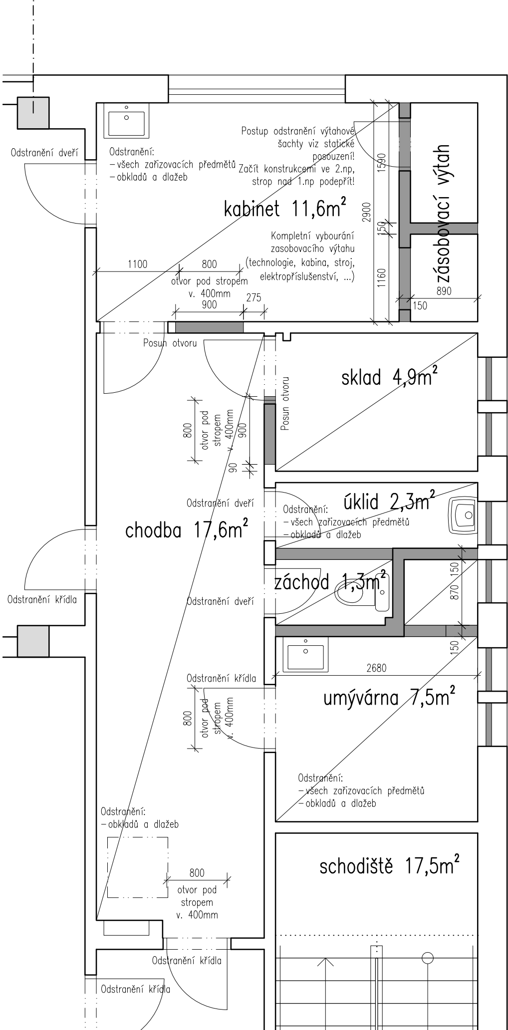
Půdorys 2.np
