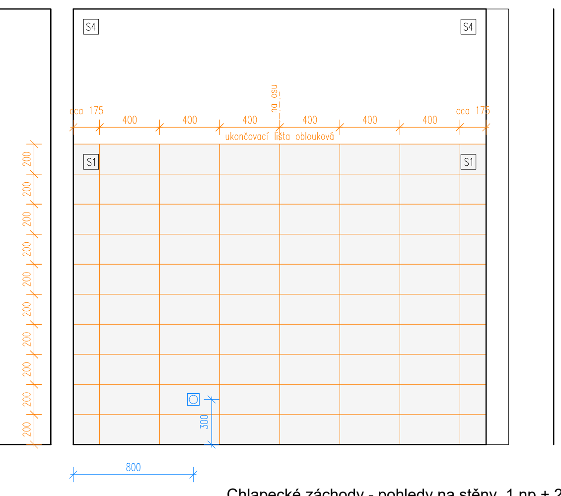
Chlapecké záchody - pohledy na stěny, 1.np + 2.np
